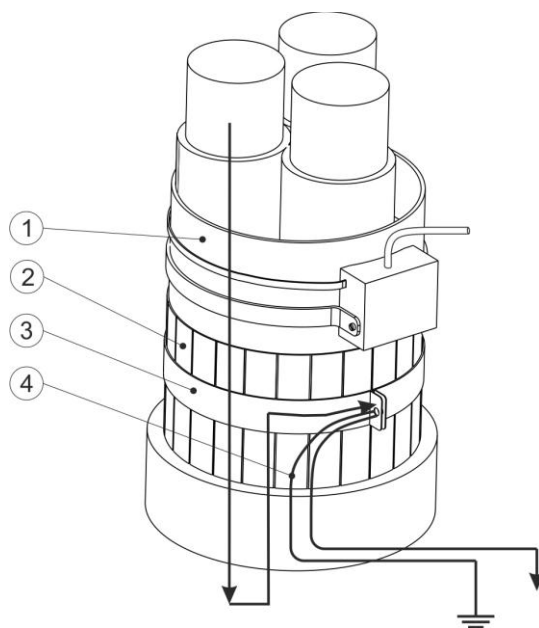
Рисунок 2.2 Датчик монтируется на экранированной части кабеля
