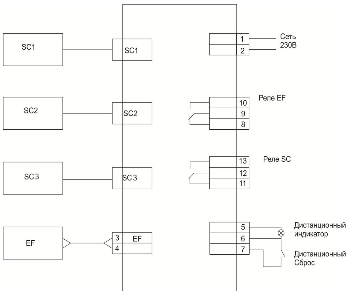
Схема подключения ИКЗ
