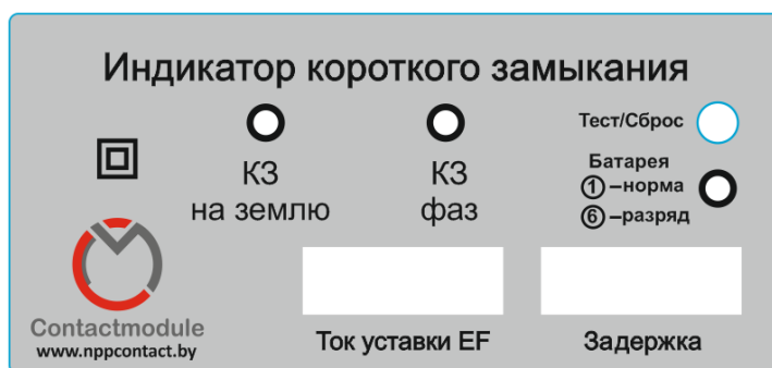
Рисунок 1.1 Передняя панель ИКЗ
